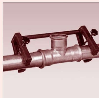
Obr. 26 Použití montážních upínadel pro „velké“ průměry Použitie montážnych upínadel pre „velké“ priemery
